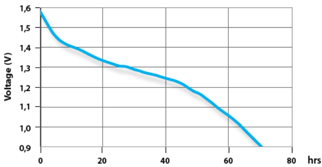
Radio 4h/d75 ohm end 0,9V
