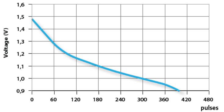
Tape 1h/d 100 mA end 0,9 volt
