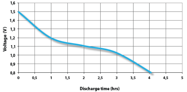
Toy 1h/d 5,1 ohm end 0,8 volt
