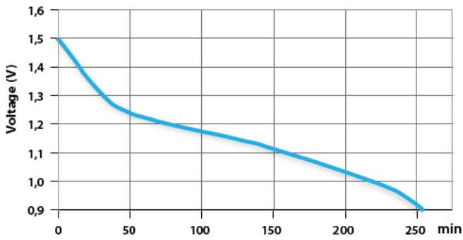
LIF 4m/h 8h/d 5,1 ohm end 0,9V
