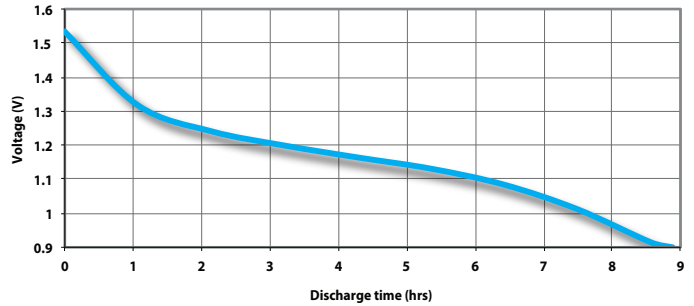
CDMD 1h/d 250 mA end 0,9 volt
