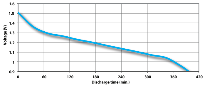
LIF 4m/h 8h/d 3,3 ohm end 0,9 volt
