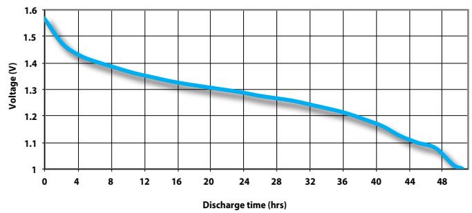
Remote Control 15s/m 8h/d 24 ohm end 1,0 volt
