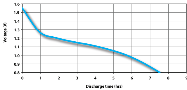
Photo flash 10s/m 1h/d 1000 mA end 0,9 volt
